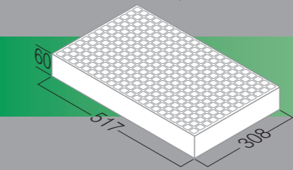
ΔΙΣΚΟΣ EPS R-286
