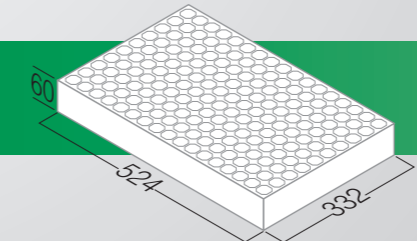
ΔΙΣΚΟΣ EPS R-170
