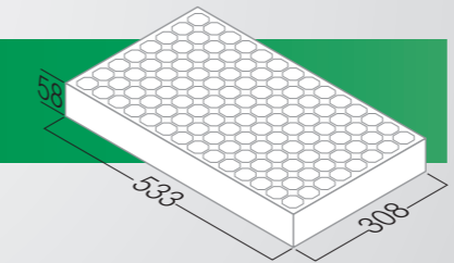
ΔΙΣΚΟΣ EPS R-112
