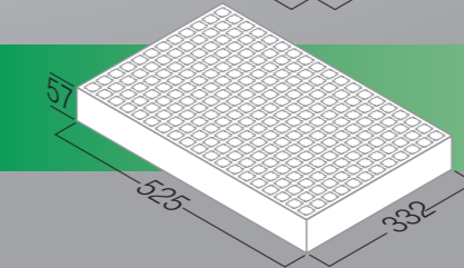
ΔΙΣΚΟΣ EPS R-228/B
