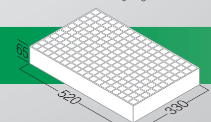
ΔΙΣΚΟΣ EPS R-198/A
