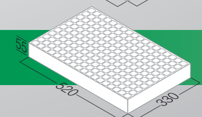
ΔΙΣΚΟΣ EPS R-198/B
